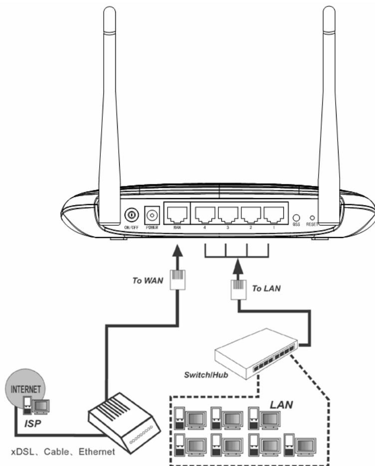
Фигура 2-1 Хардуерна инсталация на TL-WR841ND 300Mbps безжичен N рутер
